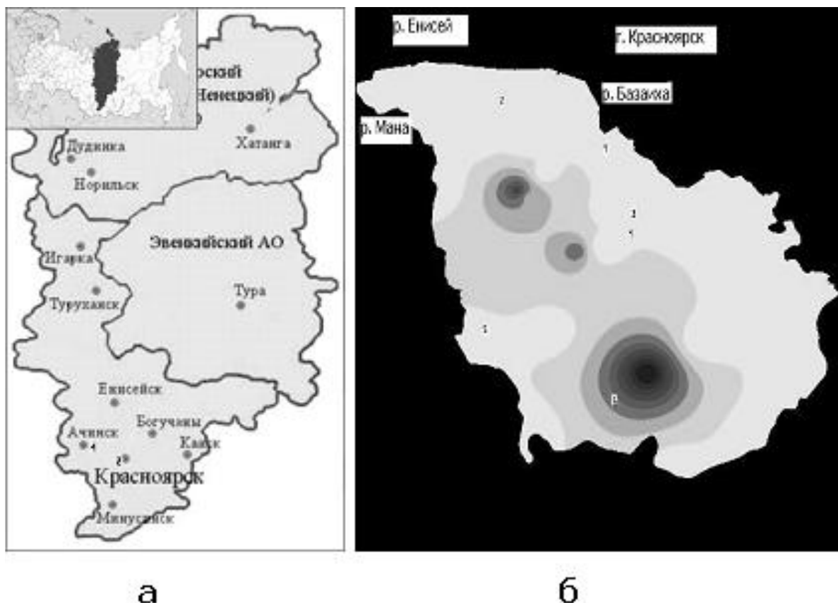
Рис. 1. Схема расположения объектов исследований: а – на территории Красноярского края: 1 – ГКЗ «Больше-Кемчугский», ПП 1; 2 – ГПЗ «Столбы», ПП 2–19; б – на территории заповедника «Столбы»: 1 – ПП 2–3, 2 – ПП 4–6, 3 – ПП 7, 4 – ПП 8–11, 5 – ПП 12–15, 6 – ПП 16–19; содержание Al в почве (мг/кг) составляет: – 0–0.39, – 0.39–0.78, – 0.78–1.17, – 1.17–1.56, – 1.56–1.95, – 1.95–2.34, – 2.34–2.73, – 2.73–3.12, – 3.12–3.51. Fig. 1. Scheme of study sites: а – in Krasnoyarsky Krai: 1 – State Complex Sanctuary «Bolshe-Kemchugskiy», study plot 1; 2 – State Nature Reserve «Stolby», study plots 2–19; б – in the State Nature Reserve «Stolby»: 1 – study plots 2–3, 2 – study plots 4–6, 3 – study plot 7, 4 – study plots 8–11, 5 – study plots 12–15, 6 – study plots 16–19. Contents of Al in soil (mg/kg) is: – 0–0.39, – 0.39–0.78, – 0.78–1.17, – 1.17–1.56, – 1.56–1.95, – 1.95–2.34, – 2.34–2.73, – 2.73–3.12, – 3.12–3.51.
