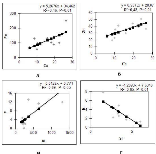
Рис. 3. Связь между содержанием в хвое усыхающих пар элементов ( p = 0.01–0.001 , n = 24 ): а – железо – кальций (Fe–Ca); б – цинк – кальций (Zn–Ca); в – фтор – алюминий (F–Al); г – никель – стронций (Ni–Sr).
