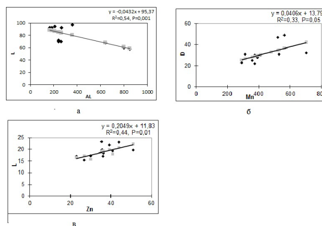
Рис. 4. Линейная регрессия между содержанием элементов и морфологическими характеристиками: а – жизненное состояние древостоев (L) – содержание в хвое алюминия (Al), б – диаметр побегов (D) – содержание марганца (Mn), в – длина хвои (L) – содержание цинка (Zn).
